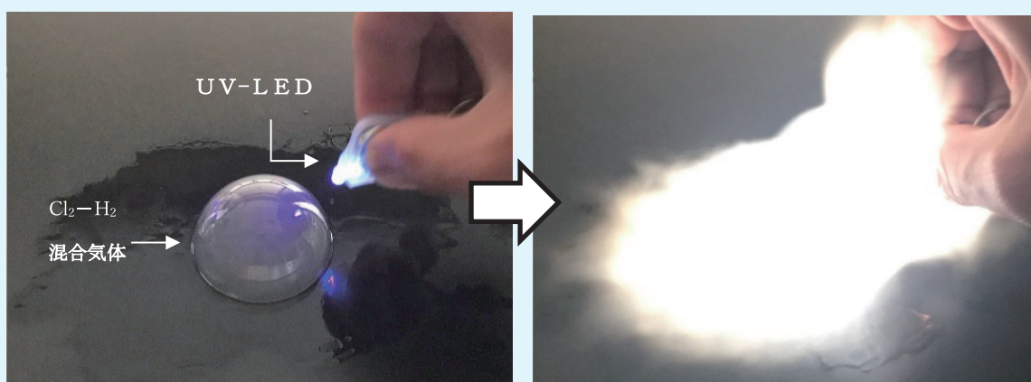
■ UV-LED による \text{Cl}_2 - \text{H}_2 混合気体の爆発 (シャボン玉法) (P435, 写真 4)
