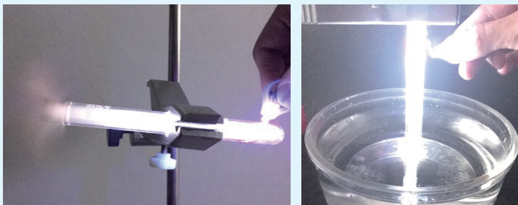
■ 試験管法による \text{Cl}_2 - \text{H}_2 混合気体の爆発 (P435, 写真 5)
