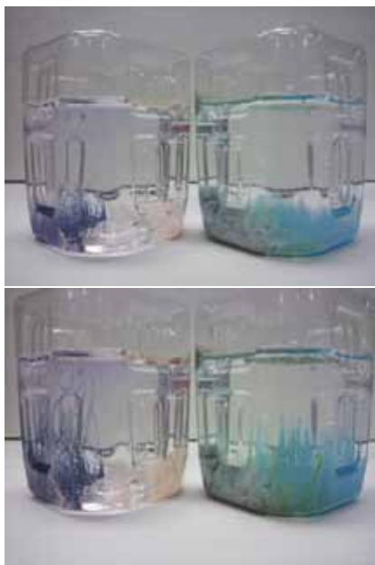
図1 金属ケイ酸塩の成長(上:5分後,下:20分後) (左)塩化コバルト六水和物,硫酸マンガン( )七水和物 (右)硫酸鉄( )七水和物,硫酸銅( )五水和物<color>
