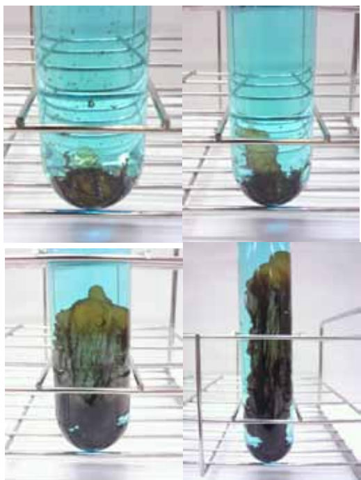
図2 ヘキサシアノ鉄( )酸銅の様子<color> (左上:5分後,右上:10分後, 左下:15分後,右下:30分後)
